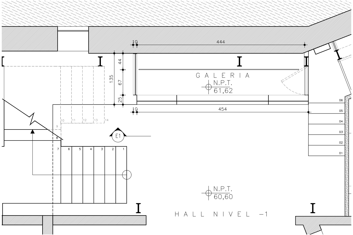
GALERIA-DIN_399 PLANTA 1 A-000 E 1:50
